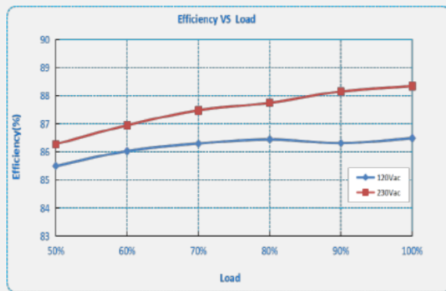
F1-040X-054 ( I_o=0.7A )
